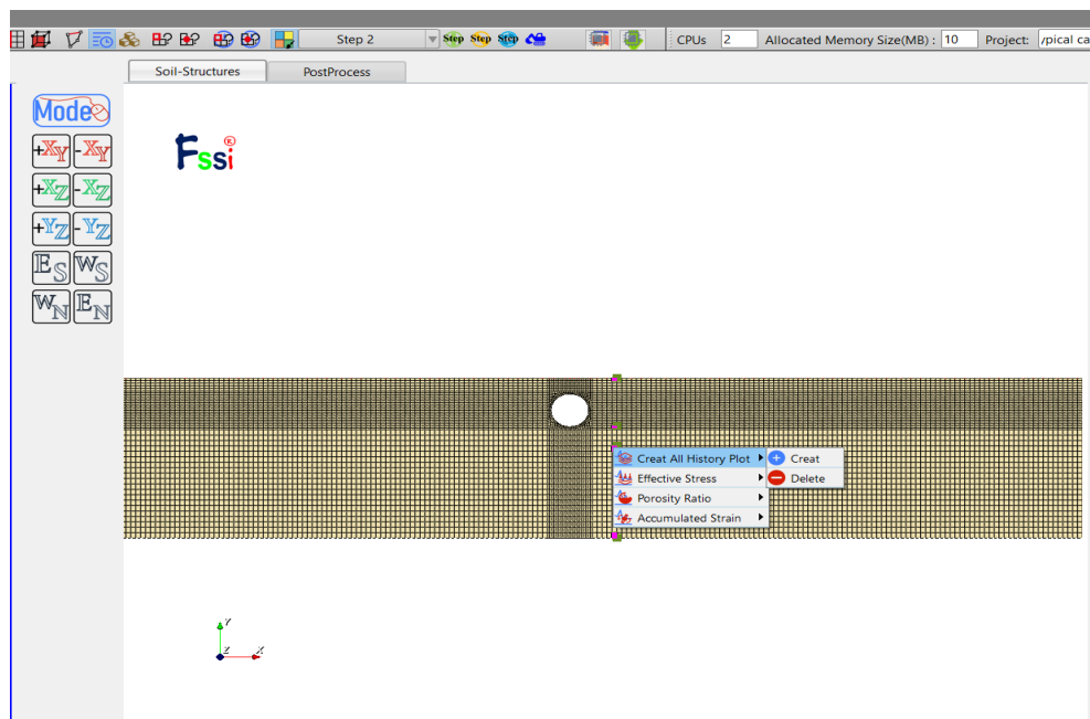
图 3-23 输出四个固体单元上的有效应力，孔隙比，应变的时程结果
