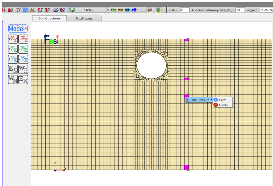
图 3-26 输出流体单元上的孔压的时程结果
