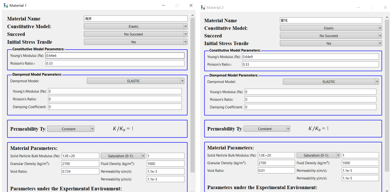
图 3-11 初始状态时海床和管线的相关属性参数
