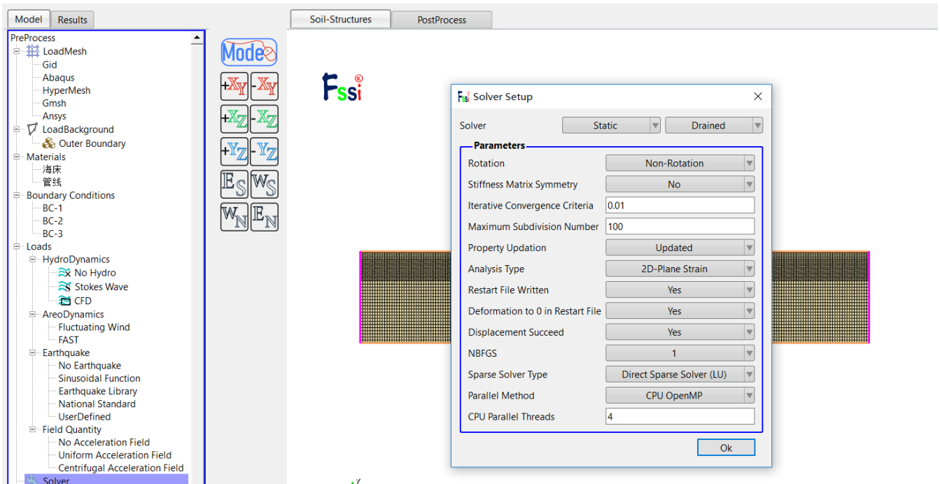
图 3-14 设置求解器的相关属性参数
