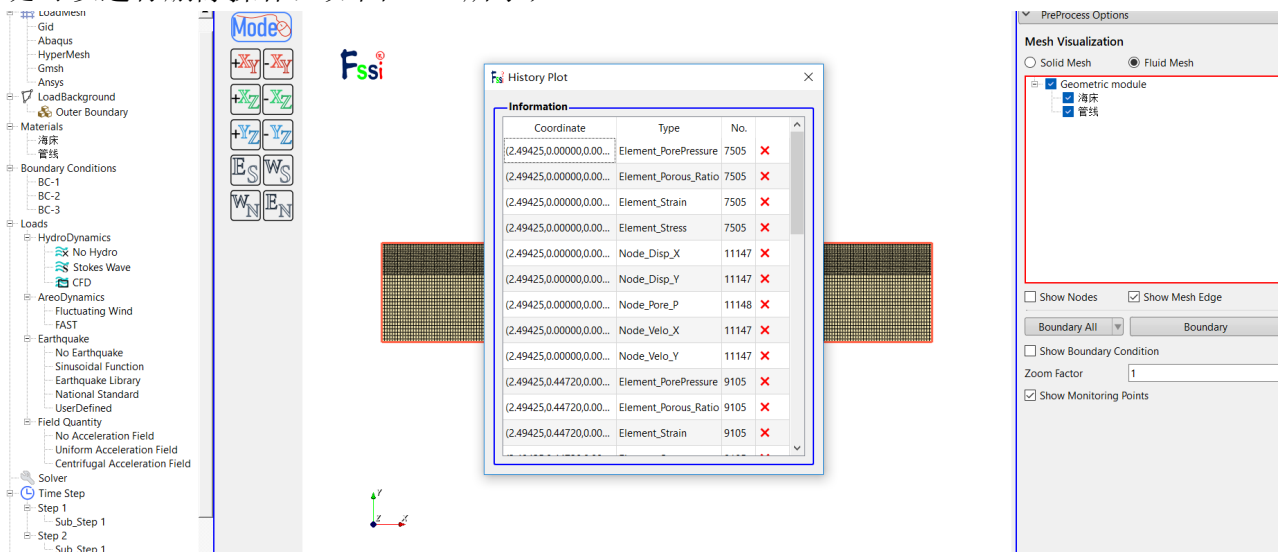
图 3-27 在前处理界面上 Model 树状菜单中的 Time History 显示已输出的时程结果列表
