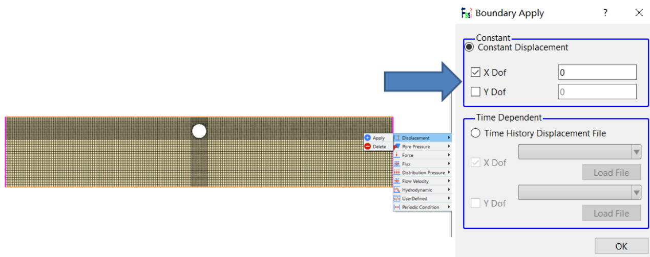
图 3-8 将左右两侧的边界设置为 X 方向位移固定
