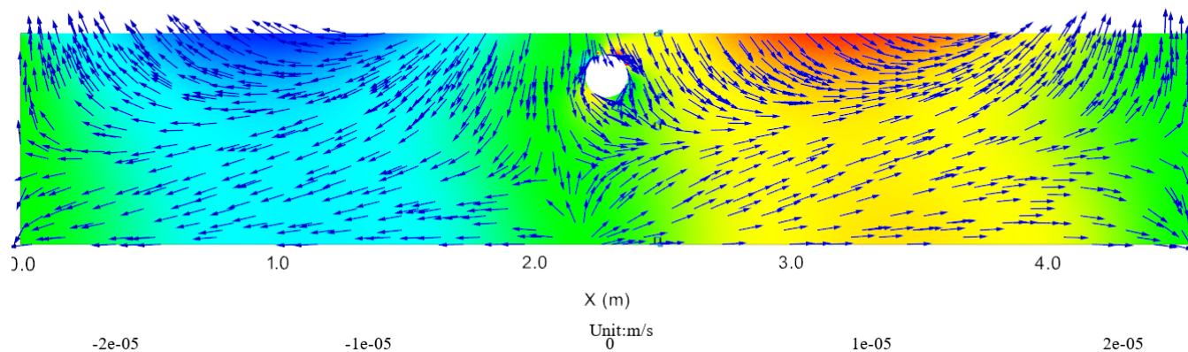
图 3-32 流线、流速图
