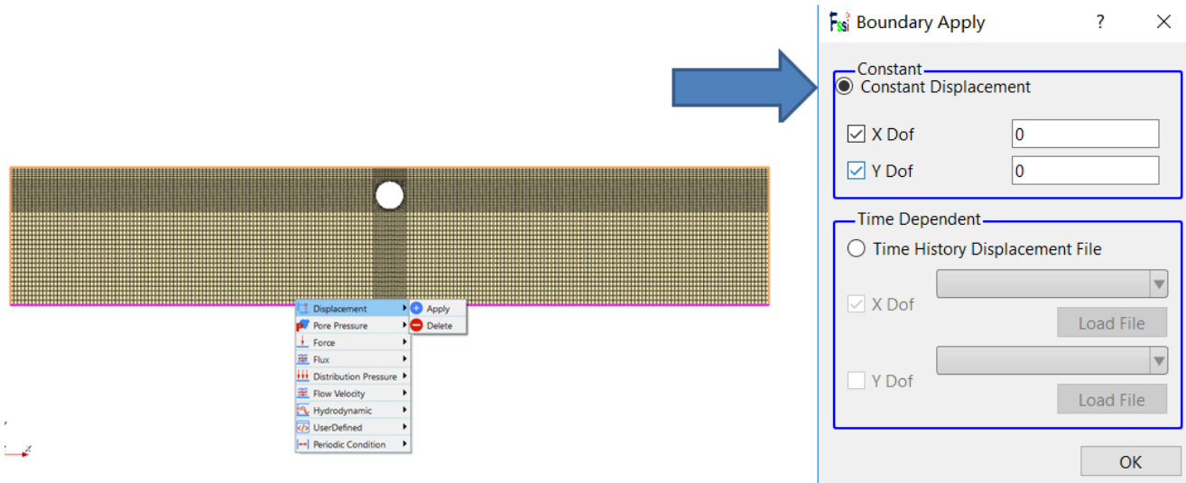
图 3-9 将底部边界设置为 X、Y 方向位移均固定
