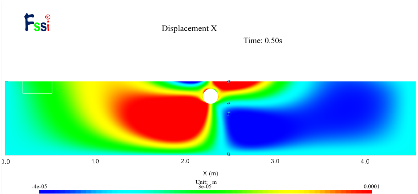
图 3-30 X 方向位移图
