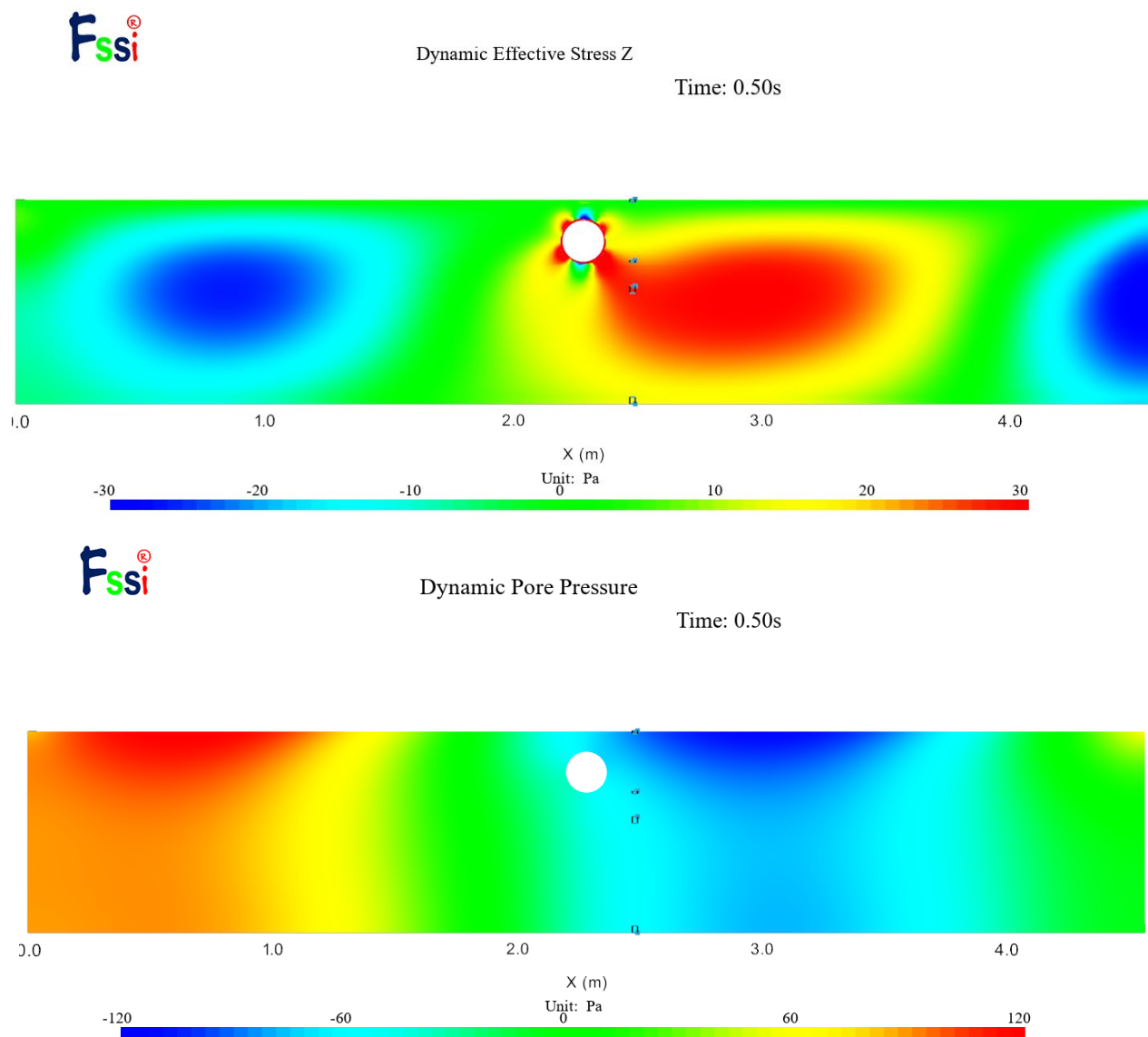
图 3-31 结果分布图
