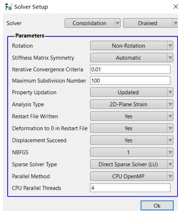
图 3-19 求解器的相关属性参数设置
