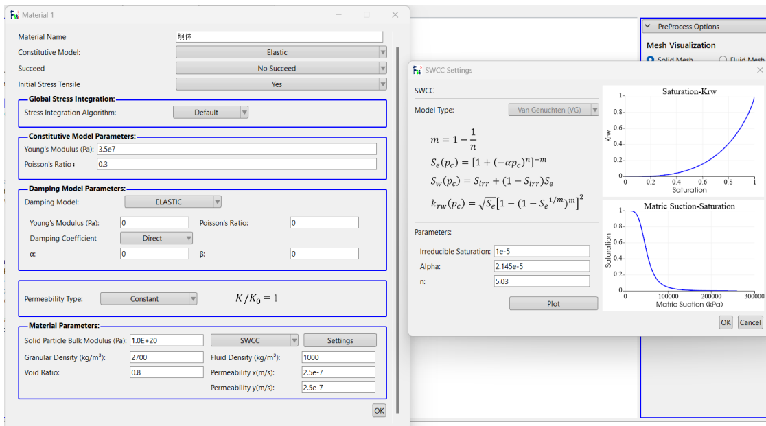
图 2-10 材料参数设置
