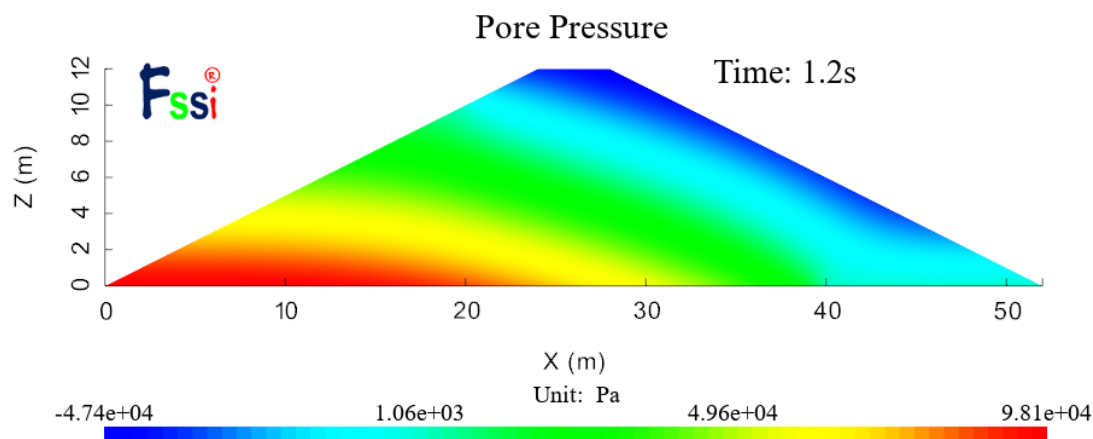
图 3-1 孔压分布图
