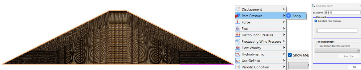
图 2-16 添加底部 0 孔压边界条件
