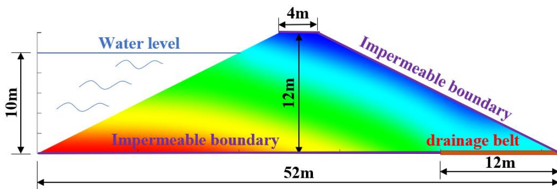
图 1-1 坝体几何形状及边界条件示意图
