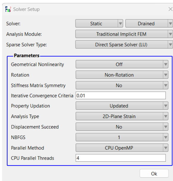
图 2-17 Step 2 求解器设置
