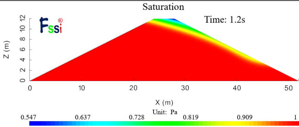
图 3-2 饱和度分布图
