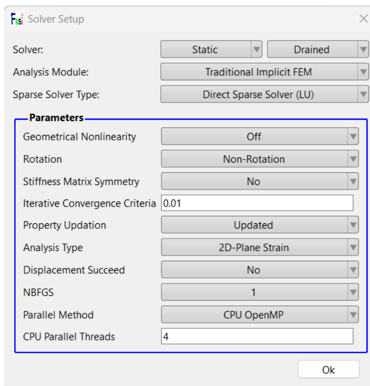
图 2-12 Step1 求解器的相关属性参数
