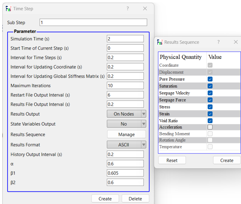
图 2-18 Step 2 时间步中各子时间步设置
