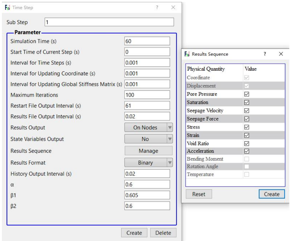
图 2.26 Step 3 时间步设置
