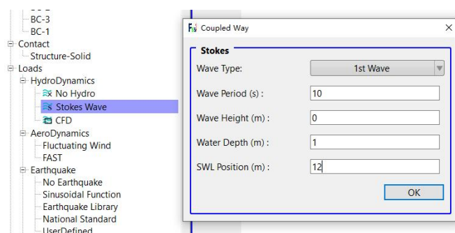
图 2.10 流固耦合方式设置界面
