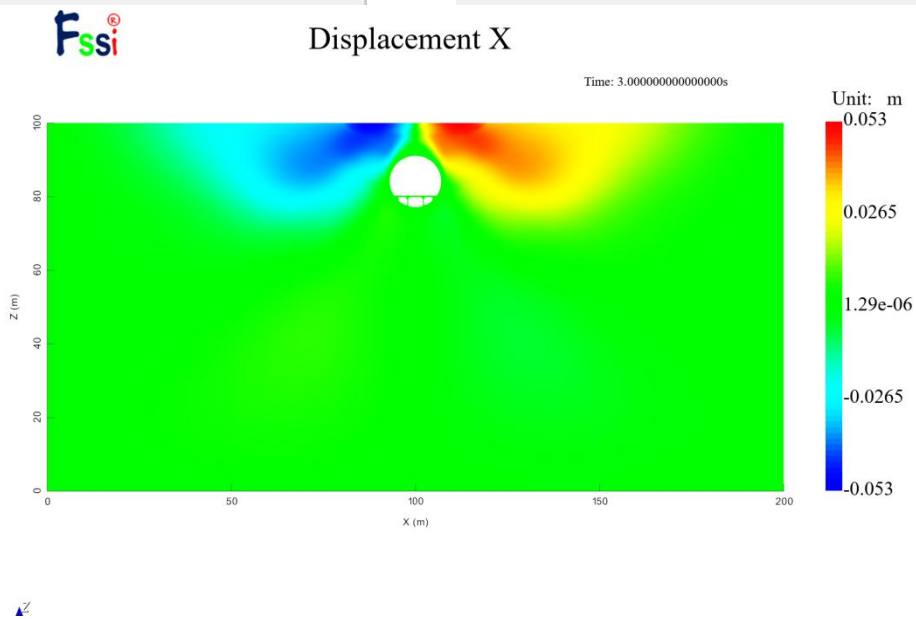
图 2-2a X方向的位移分布图（3s）
