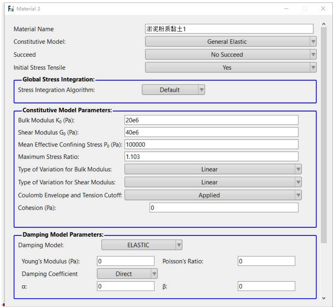
(Material 2\6\7 - 淤泥质粉质粘土 ) 图 1-13 Step 2 材料参数设置
