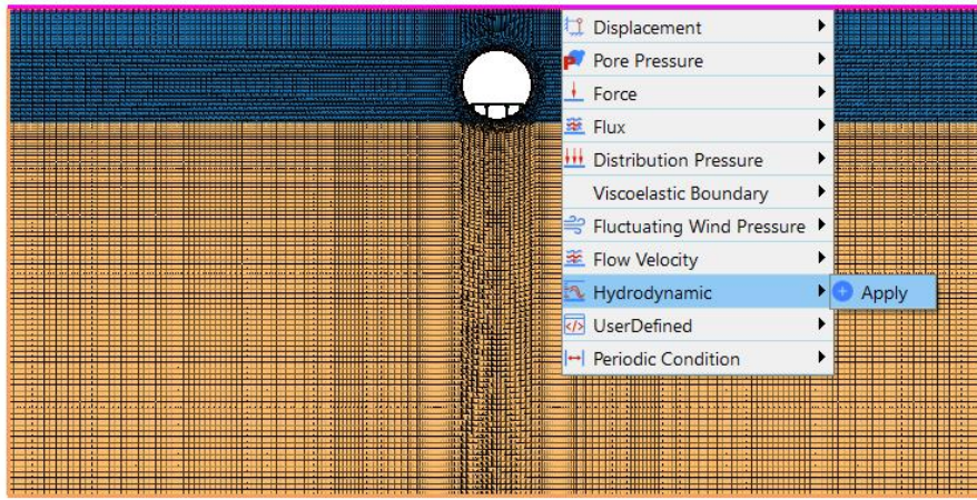
图 1-6 顶部设置水动力边界
