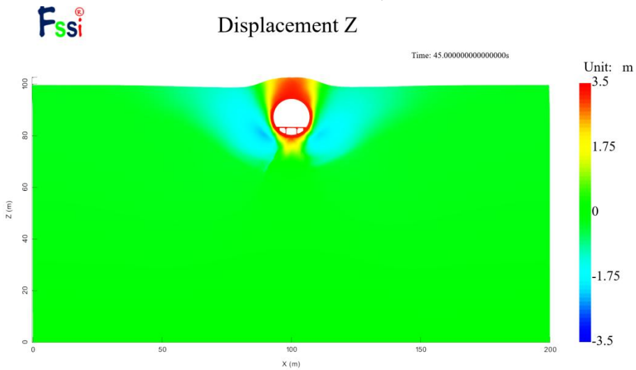
图 2-2b Z方向的位移分布图（3s）
