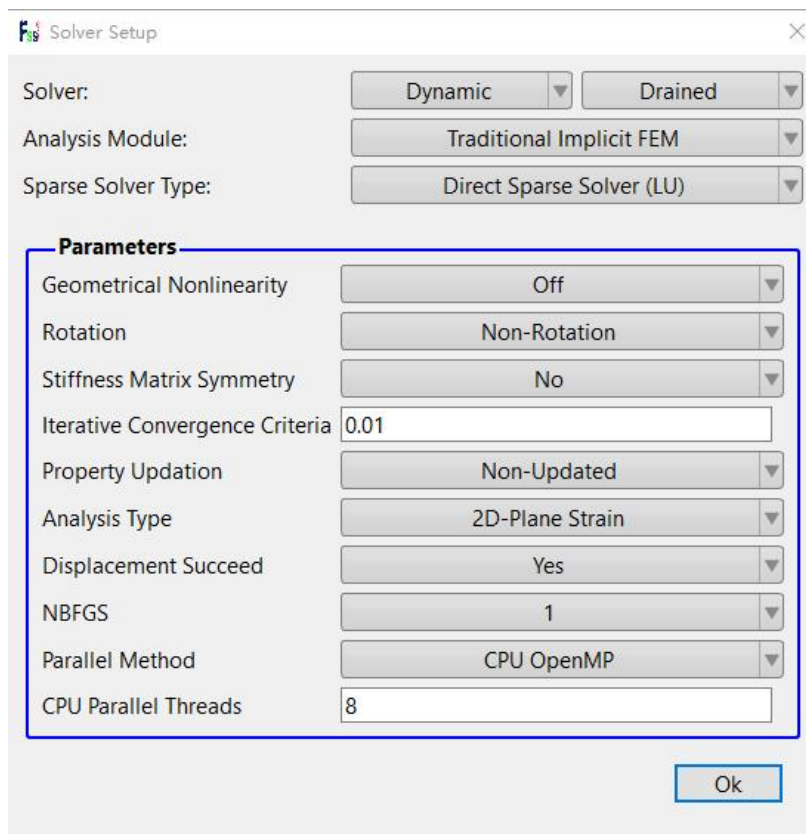
图 1-19 Step 4 求解器设置
