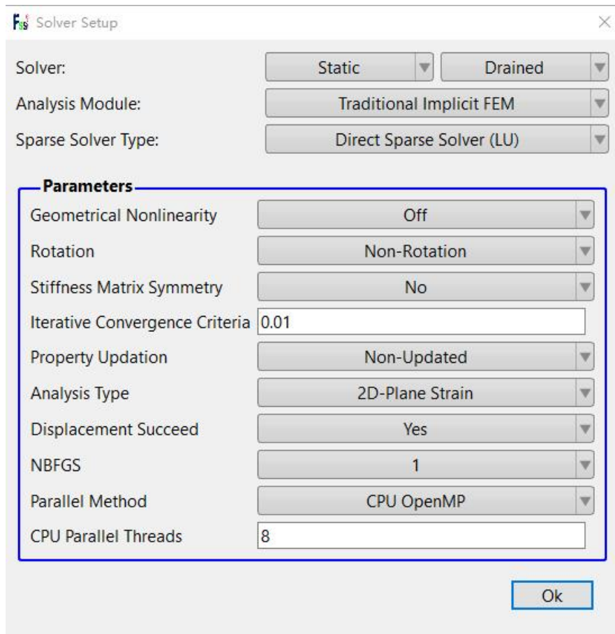
图 1-10 求解器类型及相关参数设置界面
