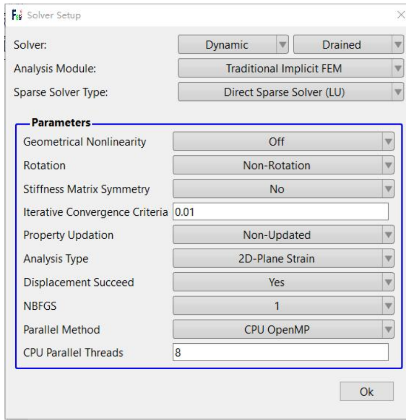
图 1-15 Step 3 求解器设置
