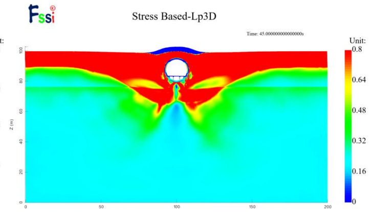
图2-3 浅埋工况各时刻液化区分布
