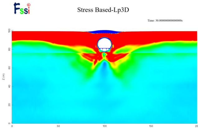
图2-3 浅埋工况各时刻液化区分布
