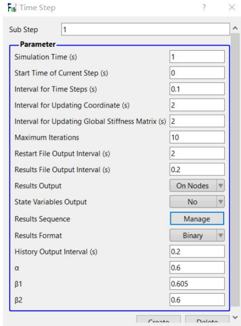
图 13-13 时间步设置
