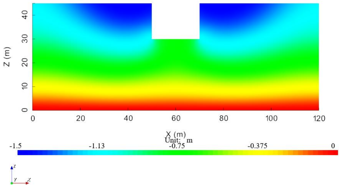
图 13-28 位移分布图
