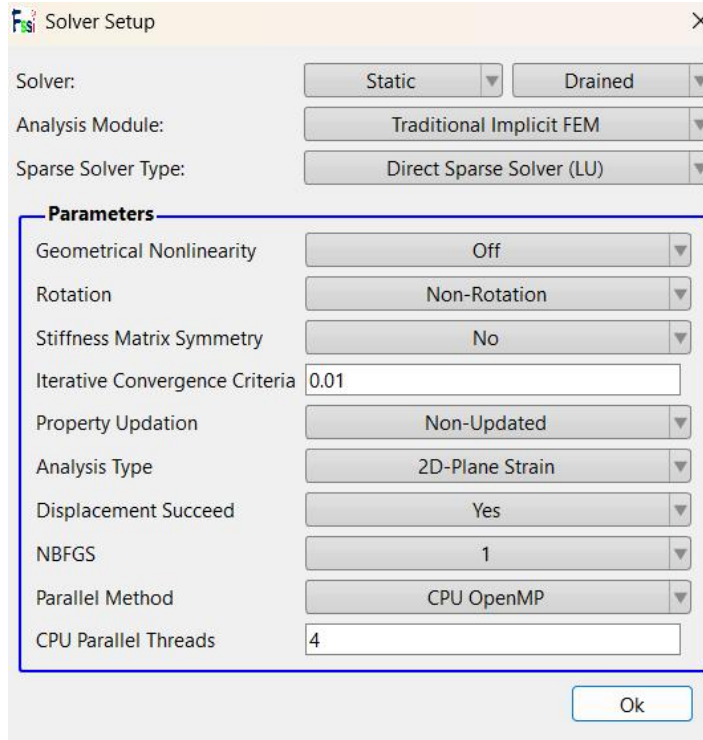
图 13-20 求解器相关参数设置
