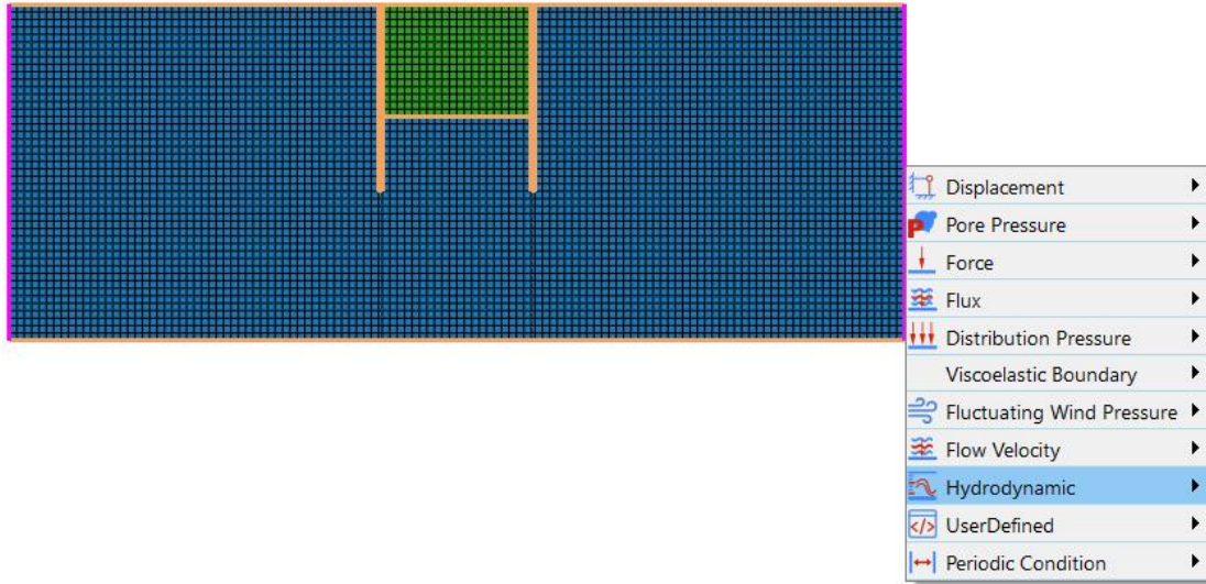
图 13-9 设置水动力边界
