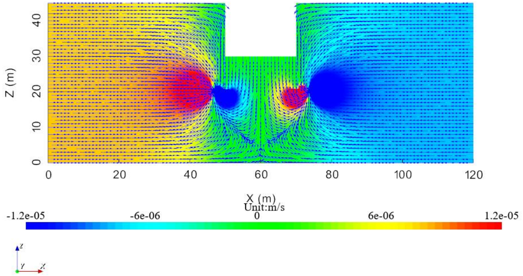
图 13-30 基坑开挖、降水流速、流线图
