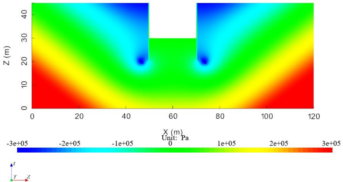
图 13-29 孔压分布图
