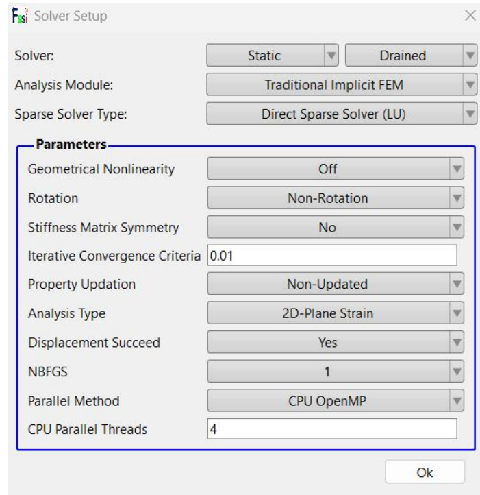
图 13-12 求解器设置
