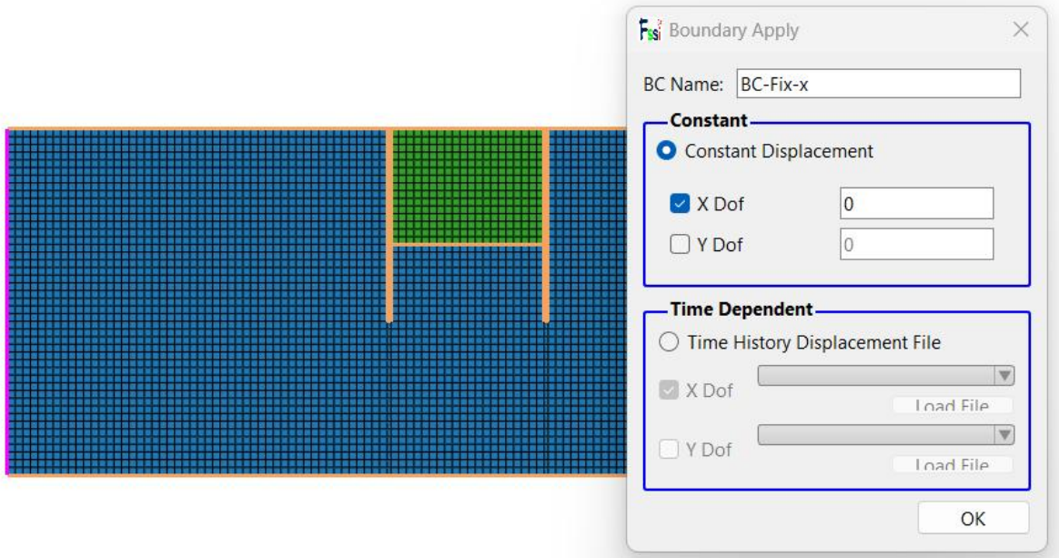
图 13-7 左右边界 X 方向位移固定
