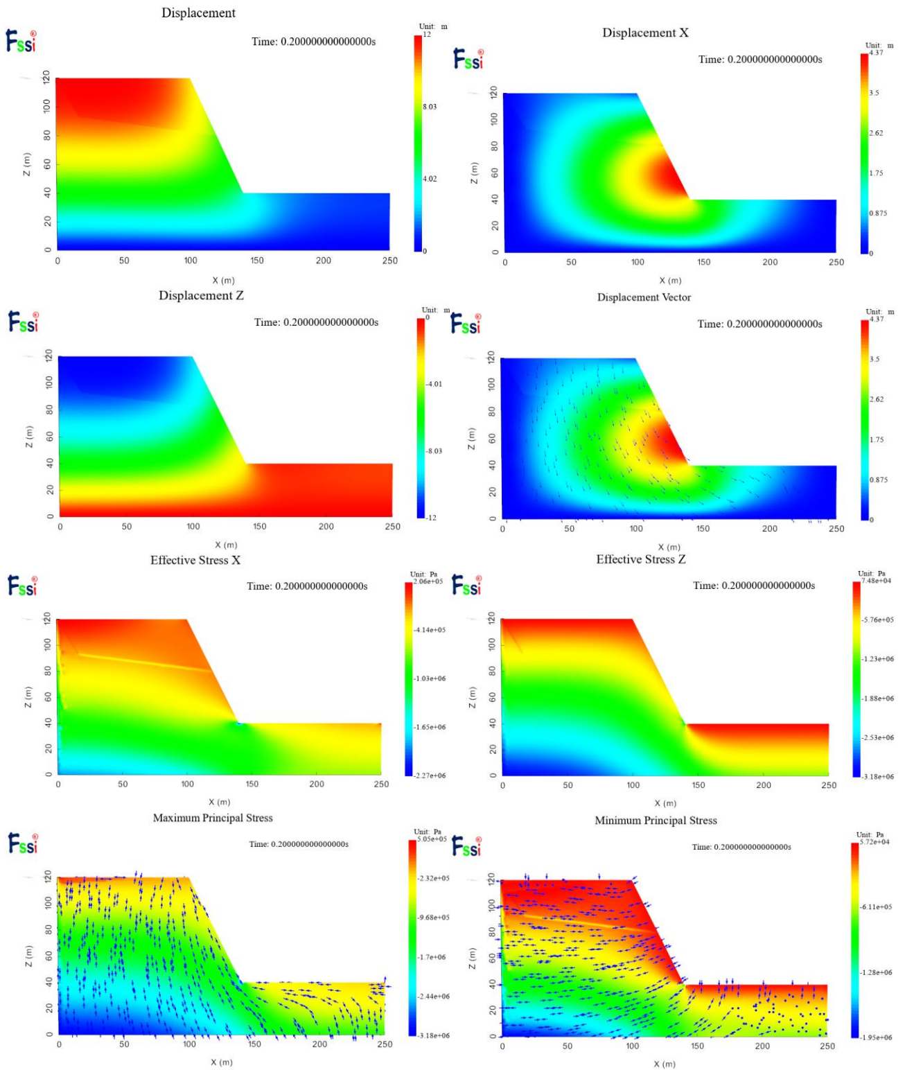
图 10-22 部分计算结果分布图
