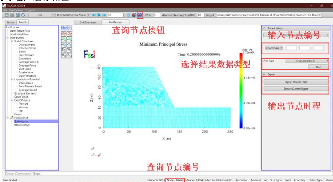
图 10-23 查询节点编号及绘制时程图
