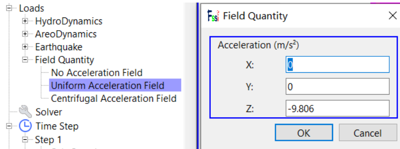
图 10-6 重力加速度设置界面
