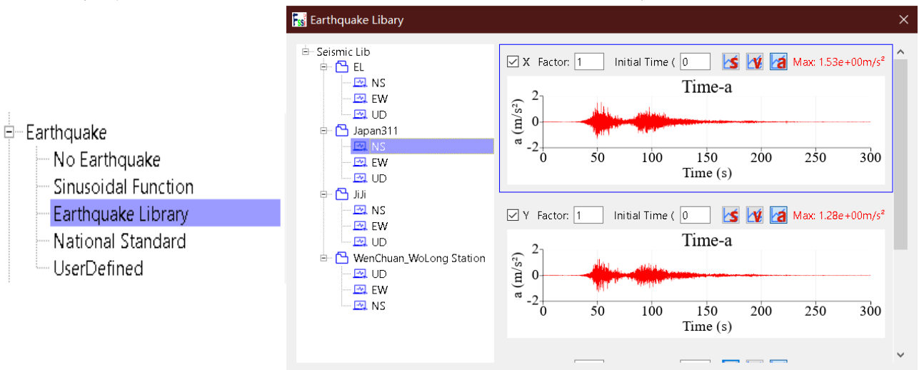
图 10-15 加载地震波及相关参数设置界面
