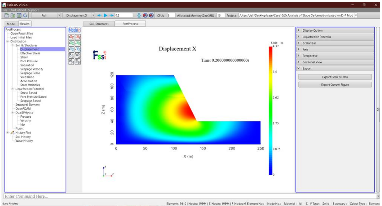
图 10-20 X 方向位移分布图
