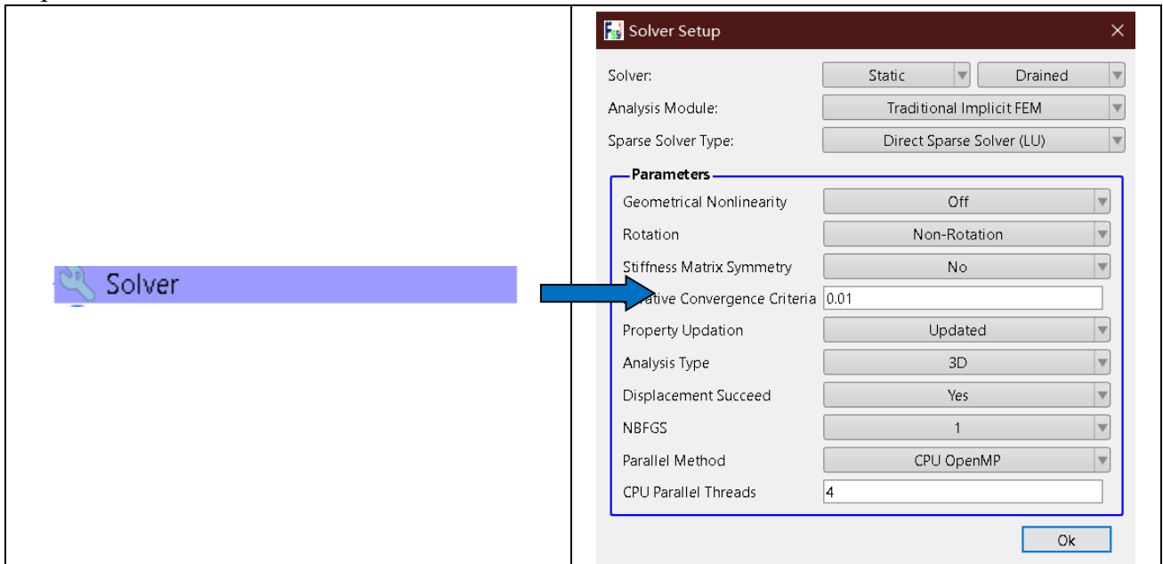
图 10-9 Step 1 求解器类型及相关参数设置界面
