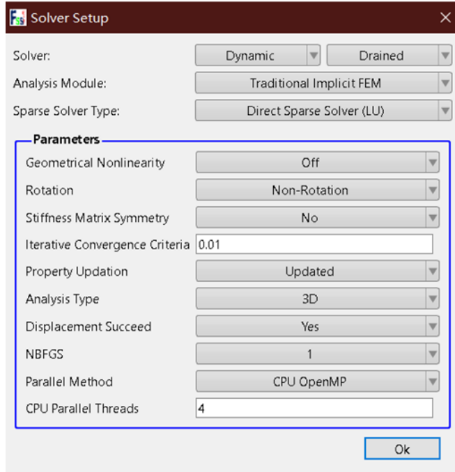
图 10-14 Step 2 求解器类型及相关参数设置界面
