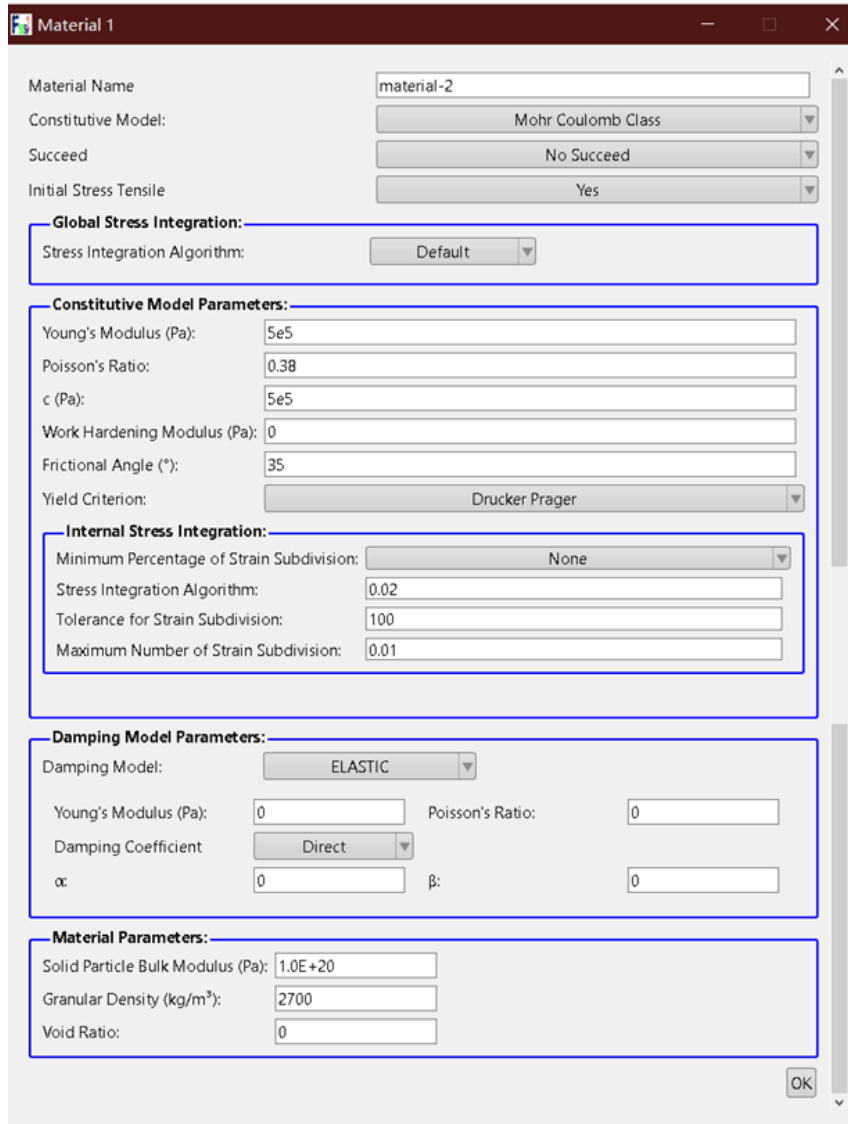
图 10-13 材料参数设置界面
